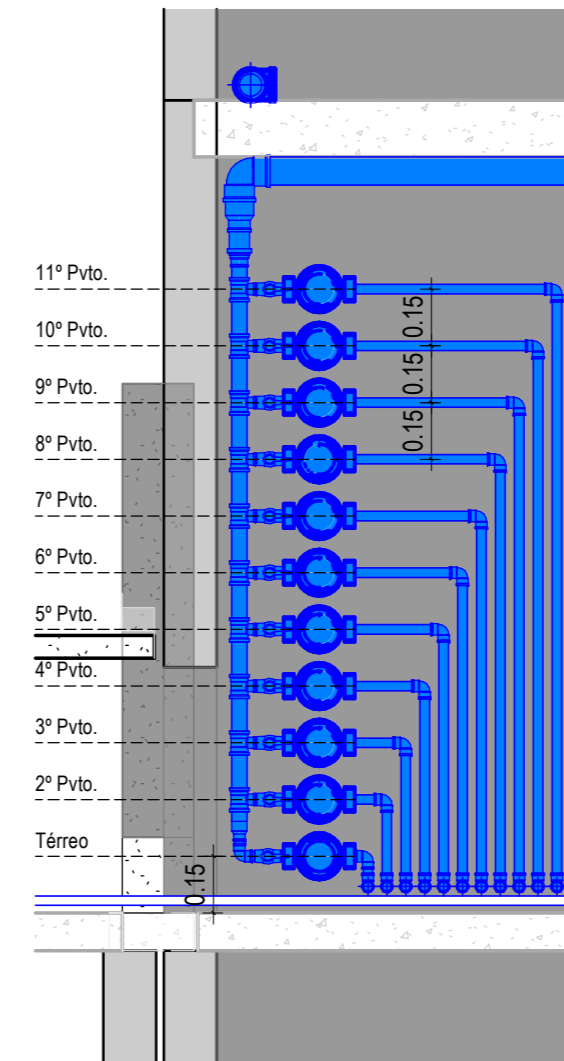
DETALHE 01 - Padrão dos medidores 1/20
