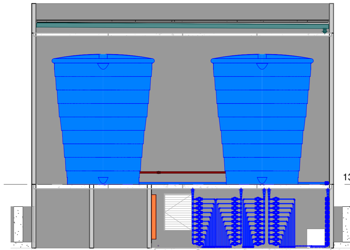
VISTA 01 - Instalações Prediais 1/75
