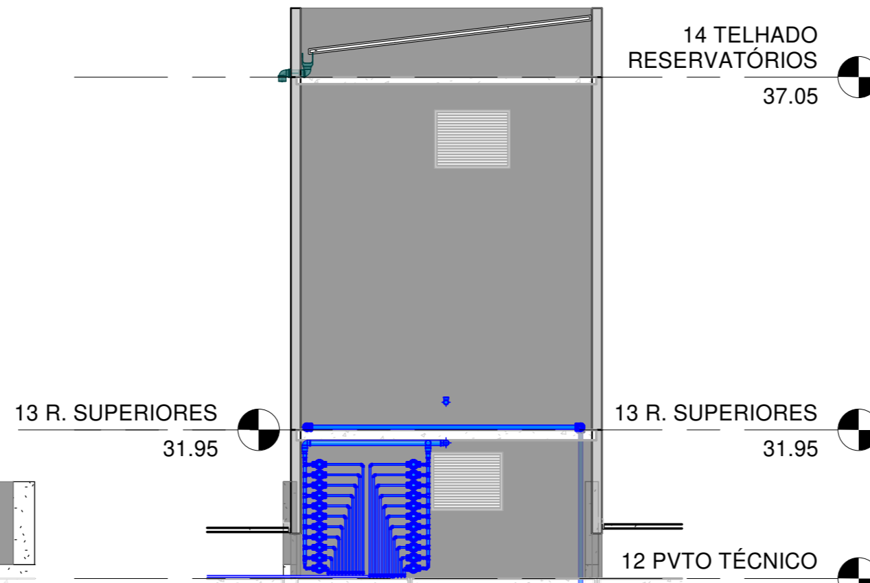
VISTA 02 - Instalações Prediais 1/75
