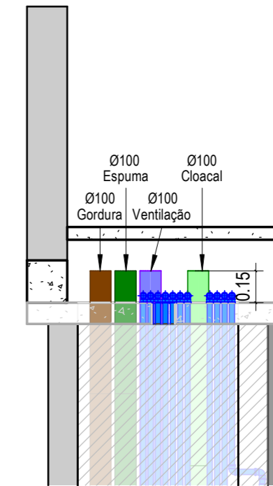
DETALHE 02 - Padrão para Terminações nos Shafts 1/25
