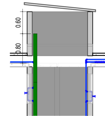
DETALHE 03 - Padrão para Terminações nos Poços 1/50
