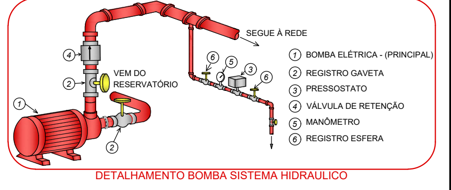
DETALHAMENTO BOMBA SISTEMA HIDRAULICO
