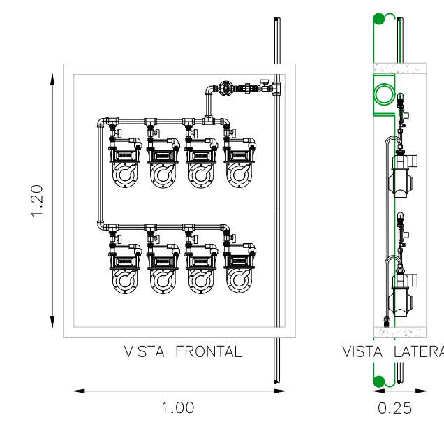
DETALHE 1 - ABRIGO DOS MEDIDORES (8 MEDIDORES) TÉRREO ESCALA: 1/25
