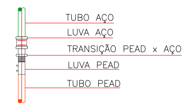
DETALHE 2 – TRANSIÇÃO PEAD x AÇO SEM ESCALA
