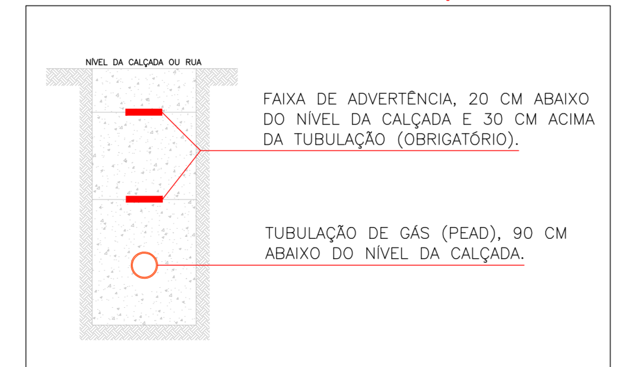
DETALHE 4 – TUBULAÇÃO EM PEAD ENTERRADA SEM ESCALA
