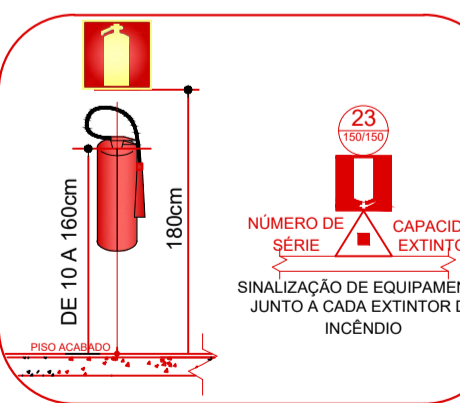
DETALHE EXTINTOR DE INCÊNDIO JUNTO A PAREDE
