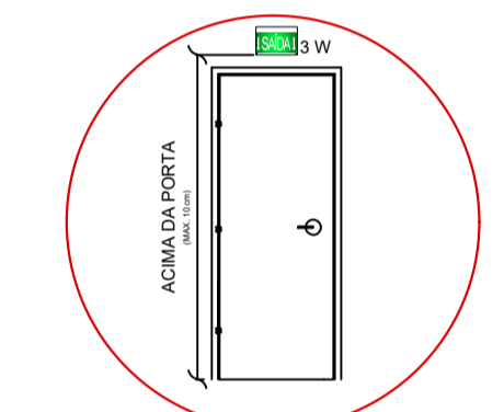
DETALHE SINALIZAÇÃO DE SAÍDA ACIMA DA PORTA (BALIZAMENTO AUTÔNOMO)
