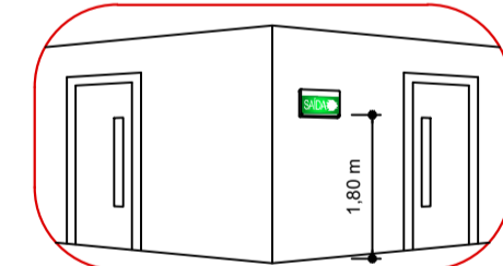
DETALHE SINALIZAÇÃO DE SAÍDA NA PAREDE
