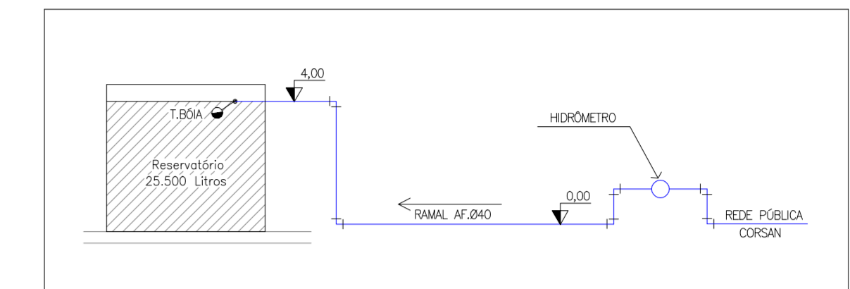
CORTE ESQUEMATICO BLOCO "A"
